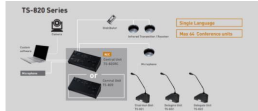
ชุดประชุมแบบไร้สาย รุ่น TS-820RC / TS-820
