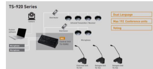
ชุดประชุมแบบไร้สาย รุ่น 920RC
